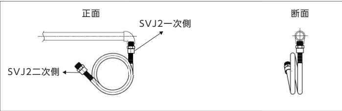
図.1 枝配管へ仮固定イメージ図 ※推奨曲げR100以上とする。
